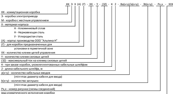
Схема составления условного обозначения коммутационной коробки электроприводов запорной и регулирующей арматуры
