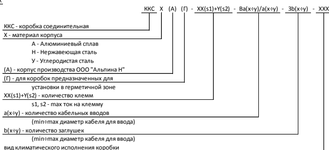
Схема составления условного обозначения коробки КИП
